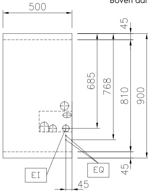
Boven aanzicht
