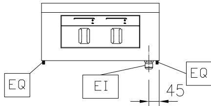
Front aanzicht
